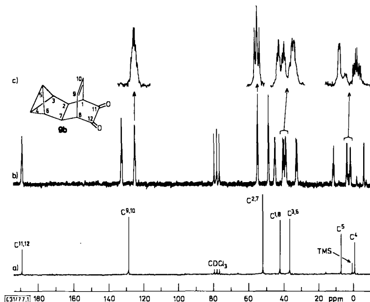
Abb. 1. 13 C-NMR-Spektrum von Pentacyclo[6.2.2.0 2,7 .0 3,5 .0 4,6 ]dodeca-9-en-11,12-dion ( 9b ) bei 22.64 MHz in CDCl 3 : a) Breitbandenkoppelt, b) protonengekoppelt, c) auf das Fünffache gedehnte Ausschnitte aus b)
